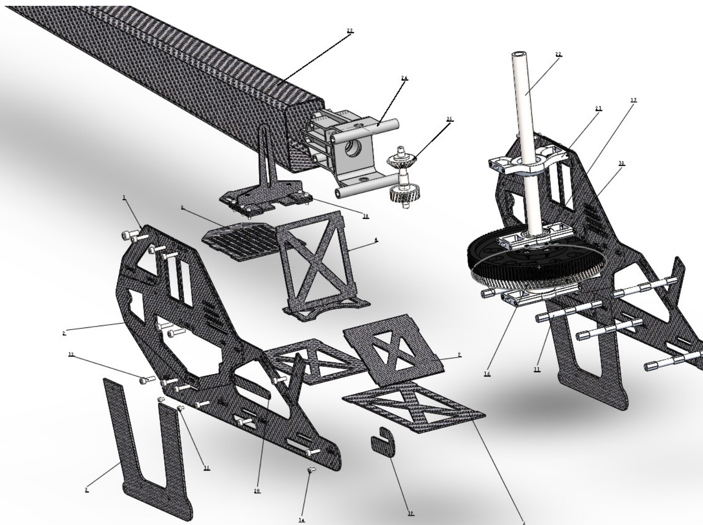
Luzifer V 2.1 Explosionszeichnung und Stückliste
